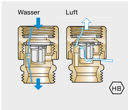
Rohrbelüfter
